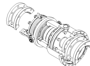
Koaxialgleitringdichtung mit Dichtungsschnellwechsel
